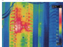
【熱画像】
