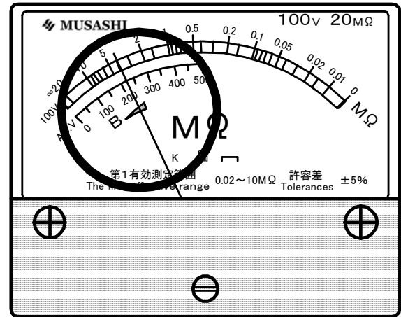
正常例 (正常な絶縁抵抗測定が できます。)
