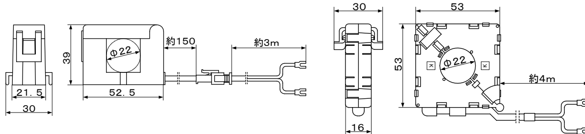
5323 MC-22 (分割電流センサ)
