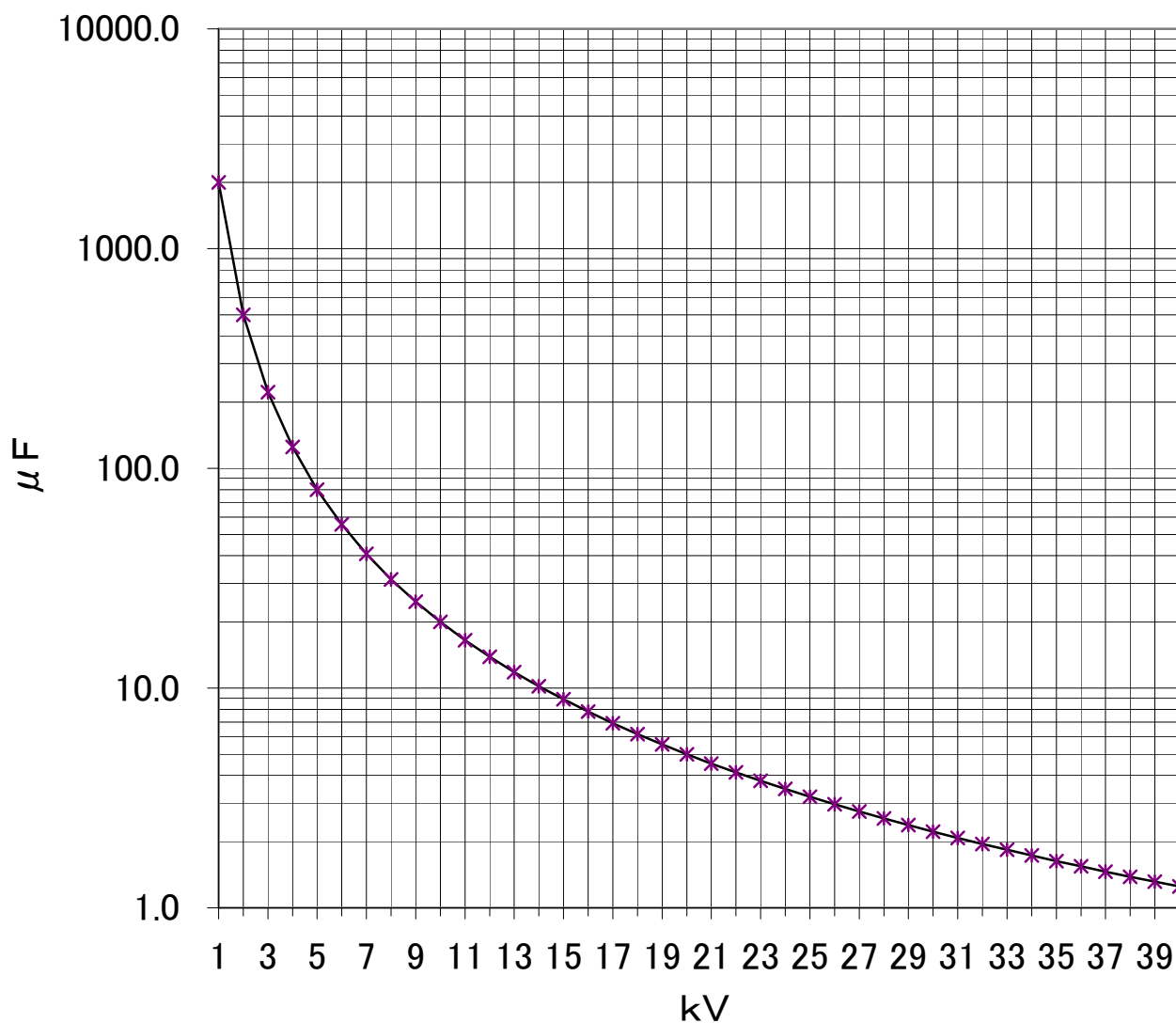
放電可能容量曲線
