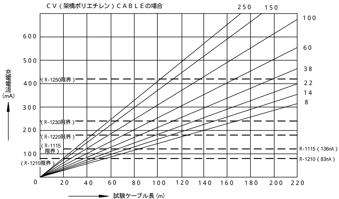
図1 6 kV用ケーブル三相一括の場合の充電電流グラフ (50 Hz)
