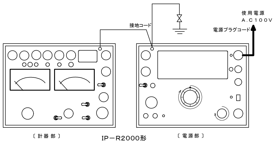
図1 試験器配置及び極性確認
