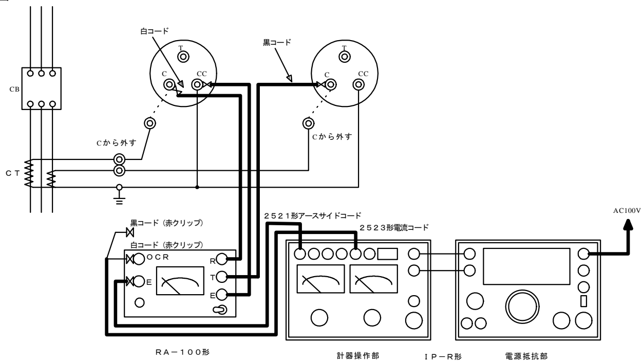
図2 動作電流特性試験
