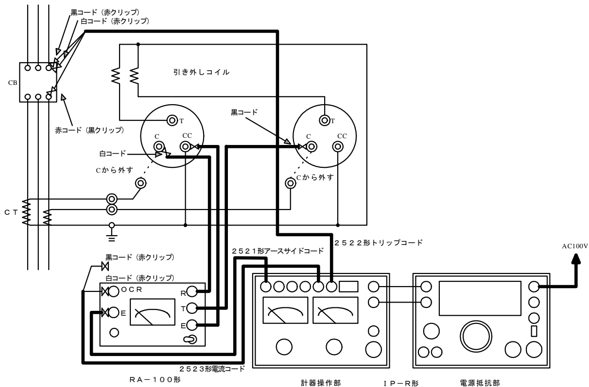
図4 CB連動試験
