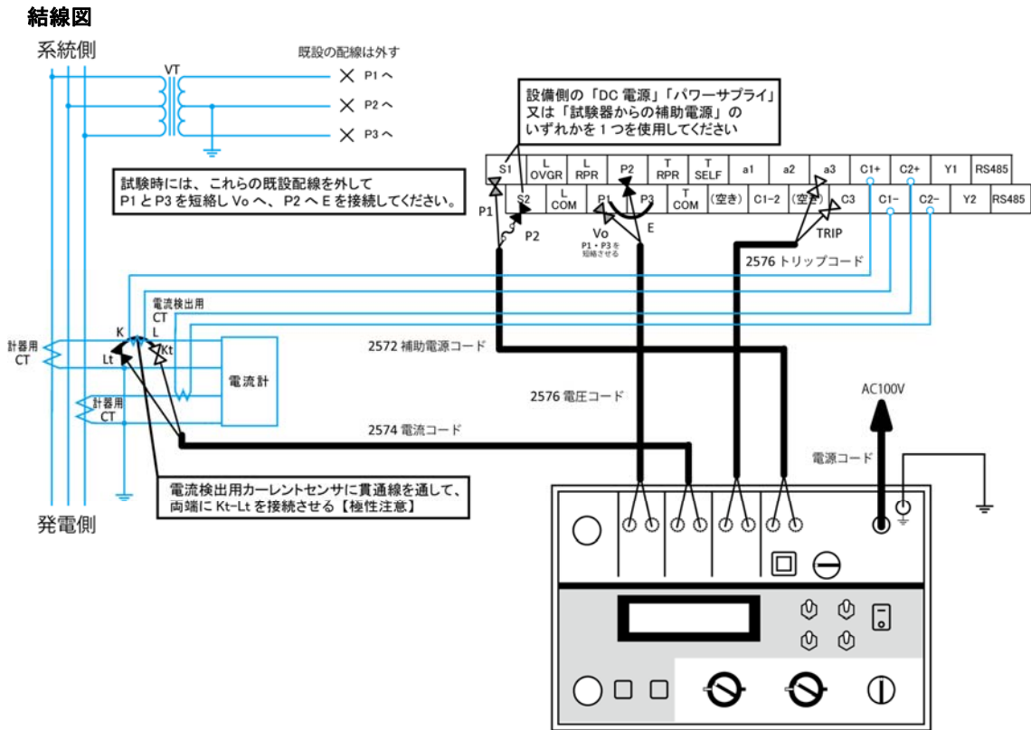
図2 逆電力継電器の配線例
