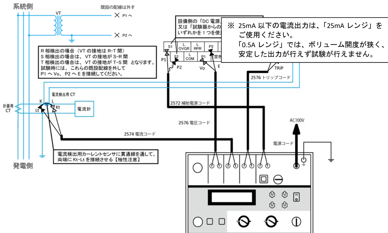
図1 逆電力継電器の配線例
