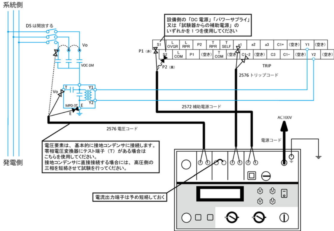
図1 地絡過電圧継電器試験の共通配線 (例: K2ZC-K2RV-NPC)
