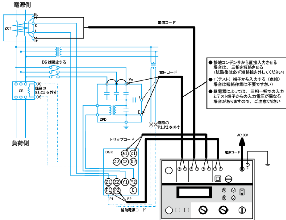
図1 地絡方向継電器試験の結線
